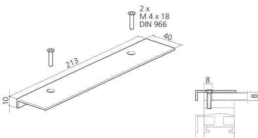
Deckleiste – End, Aluminium mit Seitenschutz Covering profile – end with side protection
