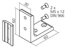
Fuß 90°, Aluminium Foot 90°
