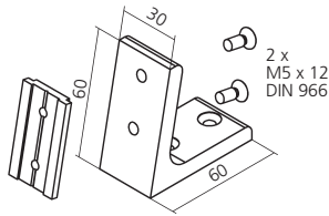
Fuß 79°, Aluminium Foot 79°
