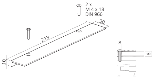
Deckleiste – End, Aluminium ohne Seitenschutz Covering profile – end without side protection
